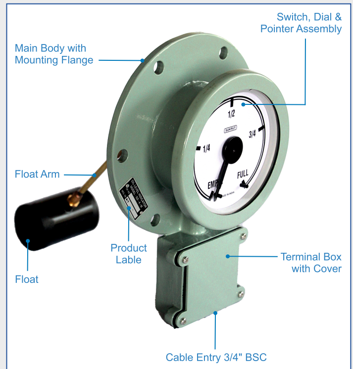
FIG. 1 SCHEMATIC
