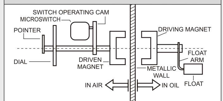
FIG. 1 SCHEMATIC
