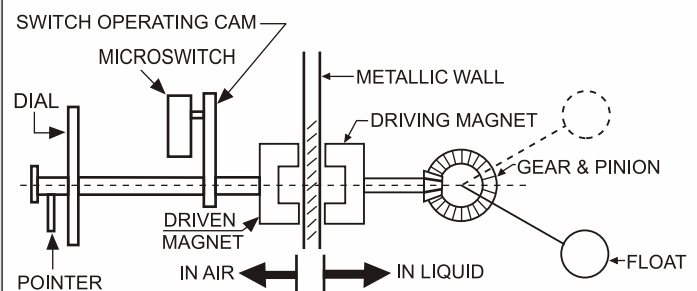
FIG. 1 SCHEMATIC
